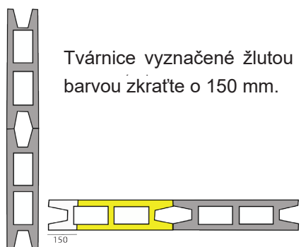
IZO 30 KLASIK
